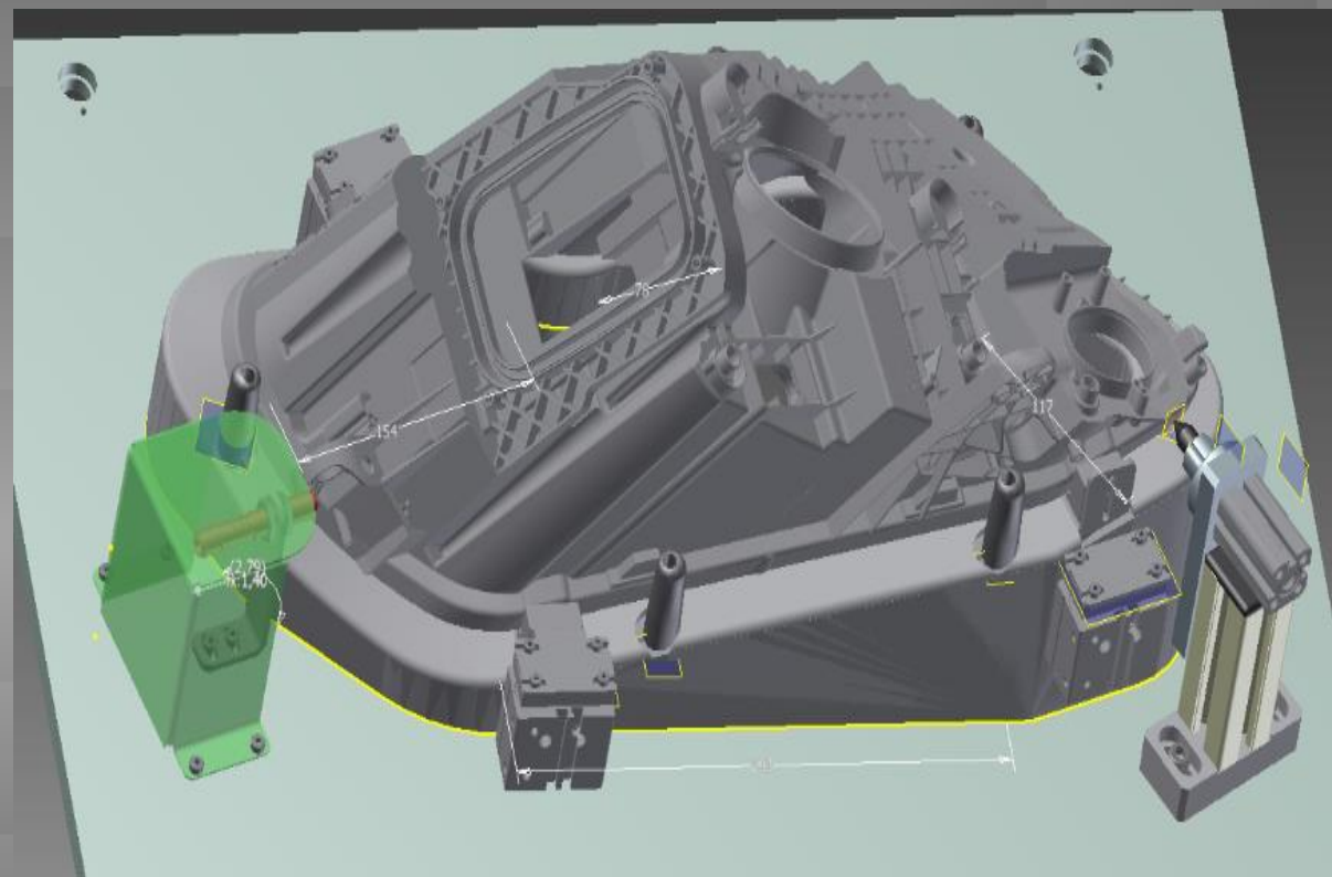
Prípravok na meranie CMM
